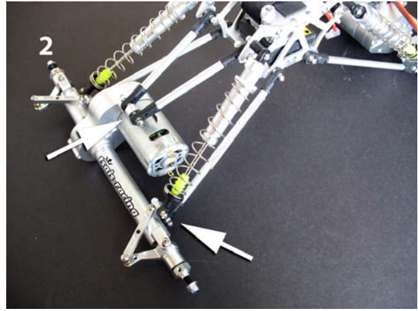
2 リア・アクスル: 示されているようにリア・アクスルの指定位置にリンクおよびショックアクソーバーを取付けてください。
