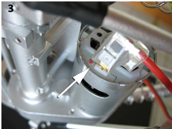
3 注意: コードを接続する際はモーターのプラスとマイナスターミナルを破損しないように注意して下さい。 ■フロントモーター: 赤(+)コードは赤印が付けられた箇所、黒(-)コードは残りもう一方のターミナルに接続します。 ■リアモーター: 黒(-)コードは赤印が付けられた箇所、赤(+)コードは残りもう一方のターミナルに接続します。(フロントとは反対)
