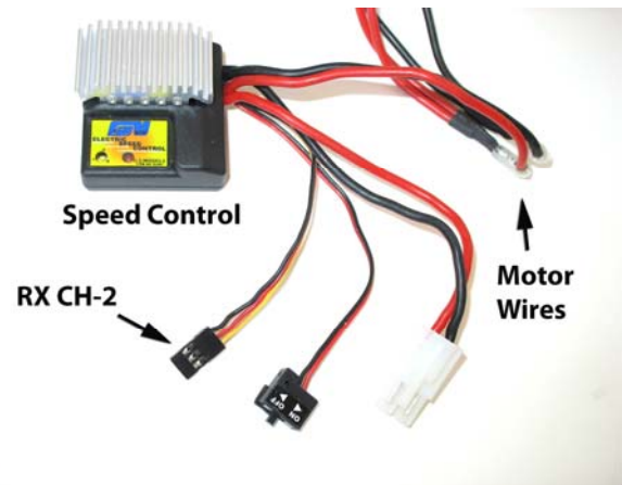
スピードコントローラー: シャーシの下甲板に取付けられています。スピードコントローラーの RX CH-2 プラグを受信機 CH2 に差し込み、モーターのコードを接続し、そして次に両面テープでシャーシの側面にスイッチを付けてください。
