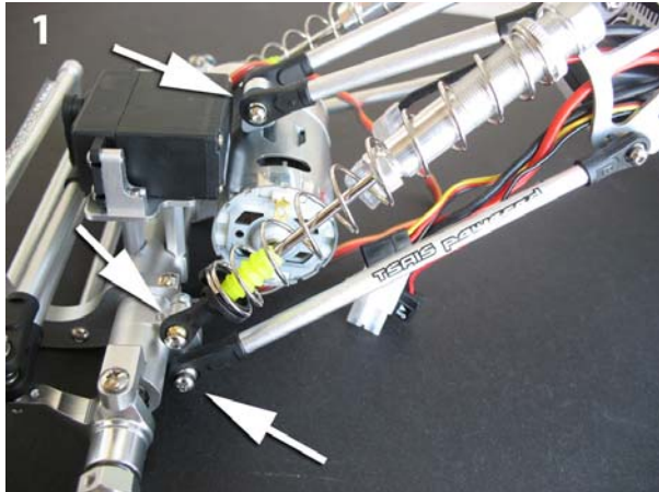
1 フロント・アクスル: 示されているようにフロント・アクスルの指定位置にリンクおよびショックアクソーバーを取付けてください。
